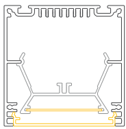
LTL70 B/H: 70x70 mm
