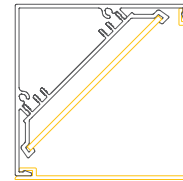
LIN70 B/H: 70x70 mm Seite
