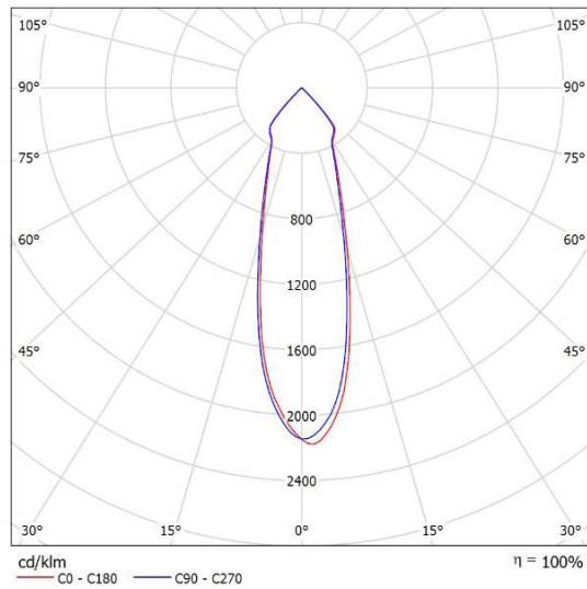
Leuchte: SML KW-D4C-15-840 Lampen: 1 x
