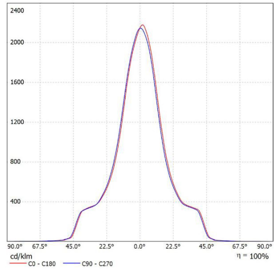
Leuchte: SML KW-D4C-15-840 Lampen: 1 x
