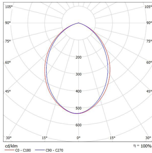
Leuchte: SML KW-D8B-25-840 Lampen: 1 x
