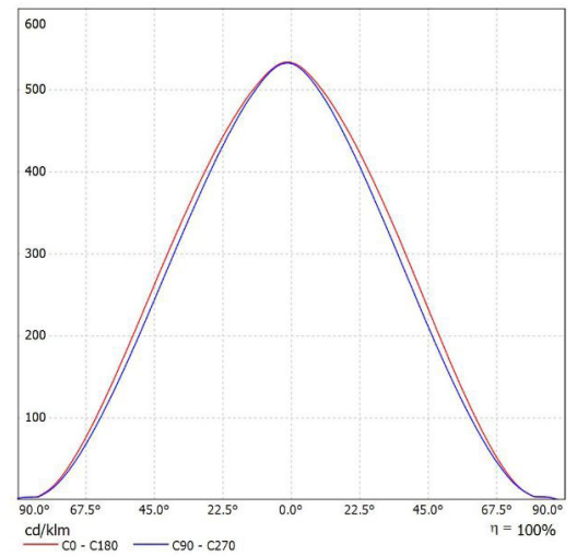
Leuchte: SML KW-D8B-25-840 Lampen: 1 x
