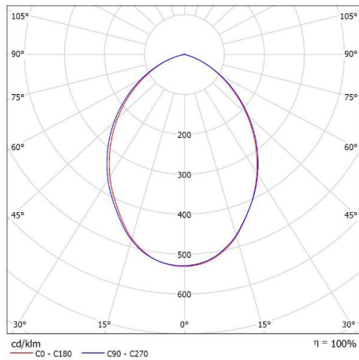
Leuchte: SML KW-D6B-25-840 Lampen: 1 x 4000K
