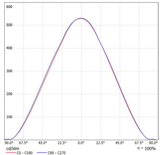
Leuchte: SML KW-D6B-25-840 Lampen: 1 x 4000K
