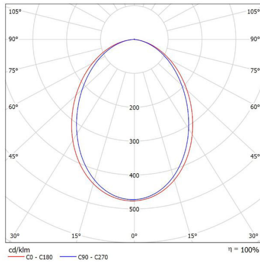
Leuchte: SML KW-D4A-25-840 Lampen: 1 x Samsung 4000K
