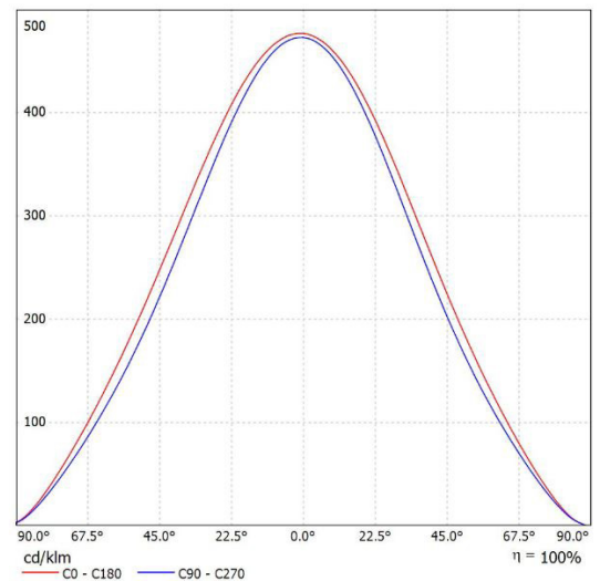
Leuchte: SML KW-D4A-25-840 Lampen: 1 x Samsung 4000K
