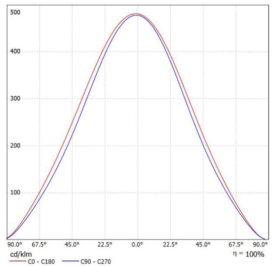
Leuchte: SML KW-D4A-20-830 Lampen: 1 x Samsung 3000K
