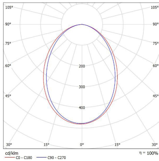
Leuchte: SML KW-D4A-20-830 Lampen: 1 x Samsung 3000K
