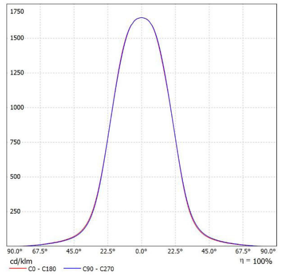
Leuchte: SML EL-EPO mini CV-4040 Lampen: 1 x 4000K
