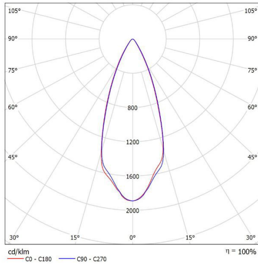
Leuchte: SML EL-EPO micro CV-4040 Lampen: 1 x 4000K
