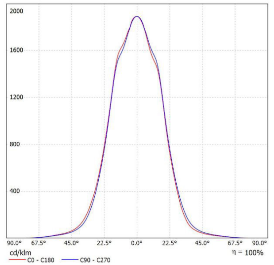
Leuchte: SML EL-EPO micro CV-4040 Lampen: 1 x 4000K
