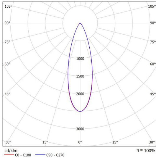
Leuchte: SML EL-EPO maxi CV-4030 Lampen: 1 x 4000K
