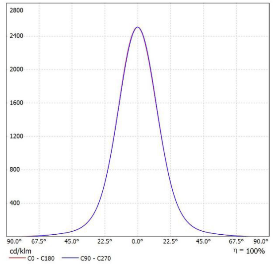
Leuchte: SML EL-EPO maxi CV-4030 Lampen: 1 x 4000K
