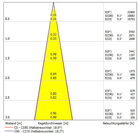
Leuchte: SML EL-E4D-08T-840-20D Lampen: 1 x CITIZEN-4000K
