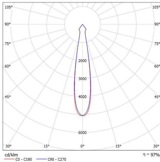
Leuchte: SML EL-E4D-08T-840-20D Lampen: 1 x CITIZEN-4000K
