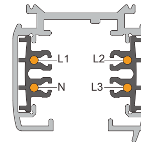
3-phasen Stromschiene
