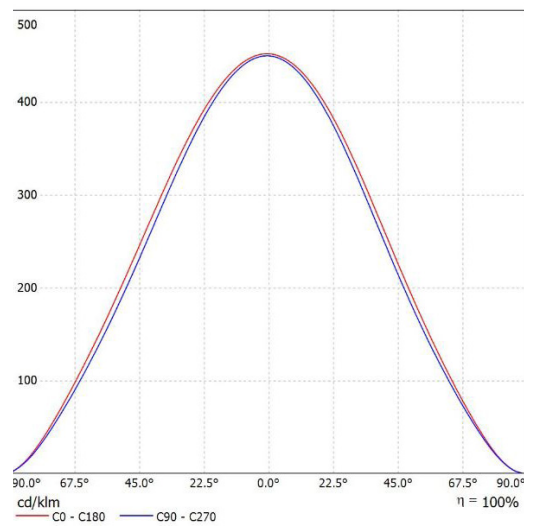
Leuchte: SML KW-D6A-32-830 ampen: 1 x Samsung 3000K
