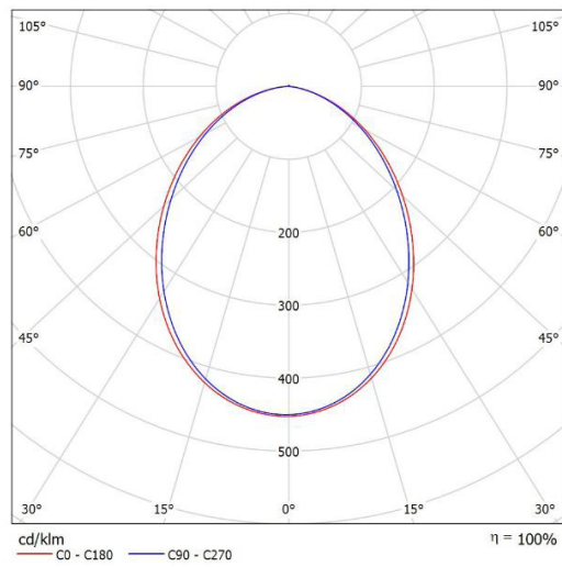
Lampen: 1 x Samsung 3000K
