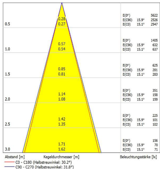
Leuchte: SML EL-G50-R5-827-36D Lampen: 1 x LUMINUS-2700K
