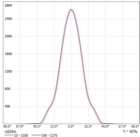
Leuchte: SML EL-G50-R5-827-36D Lampen: 1 x LUMINUS-2700K
