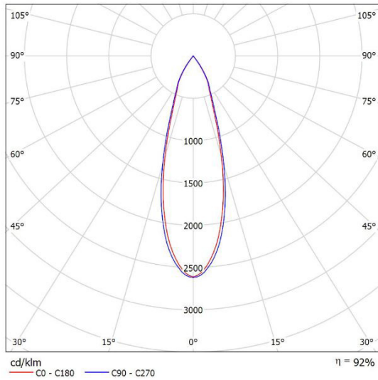
Leuchte: SML EL-G50-R5-827-36D Lampen: 1 x LUMINUS-2700K
