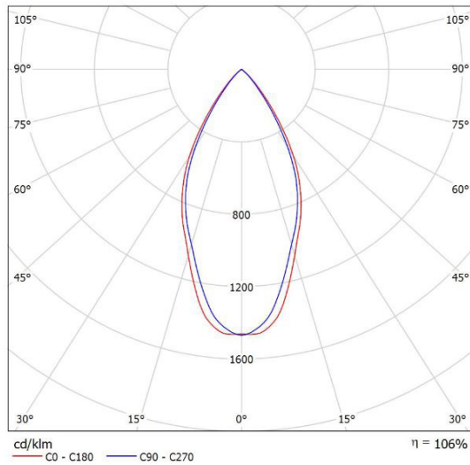
Leuchte: SML EL-CITA-30T-940-50 Lampen: 1 x CITIZEN-4000K
