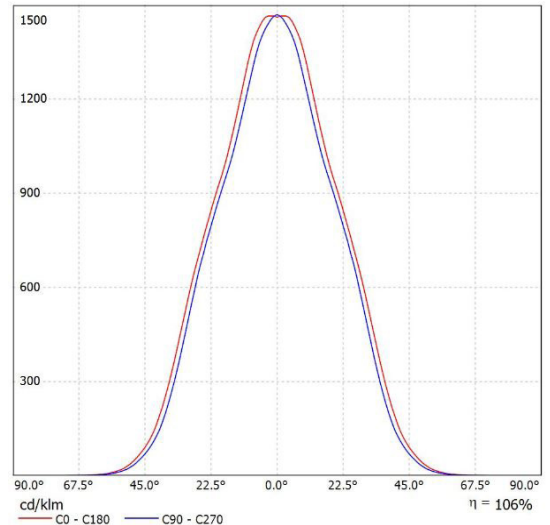
Leuchte: SML EL-CITA-30T-940-50 Lampen: 1 x CITIZEN-4000K
