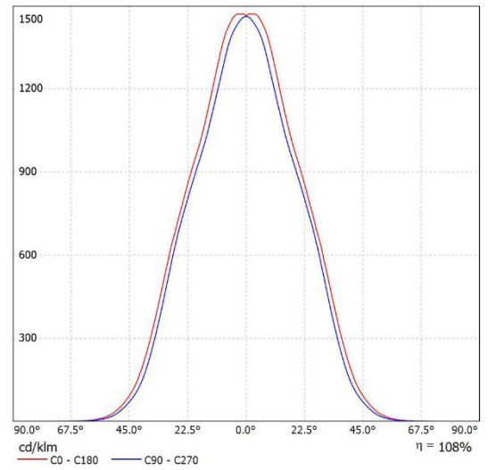
Leuchte: SML EL-CITA-30T-840-50 Lampen: 1 x CITIZEN-4000K
