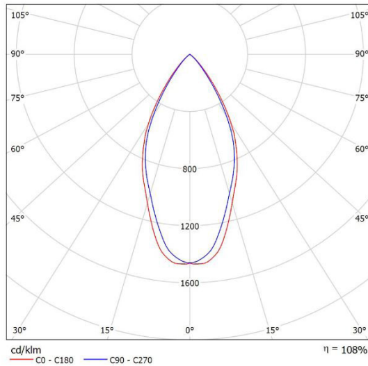
Leuchte: SML EL-CITA-30T-840-50 Lampen: 1 x CITIZEN-4000K
