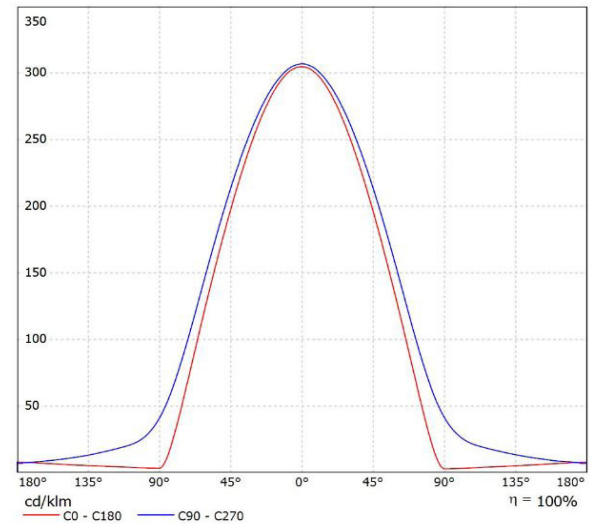
Leuchte: SML SH-A65F4-50-4F Lampen: 1 x
